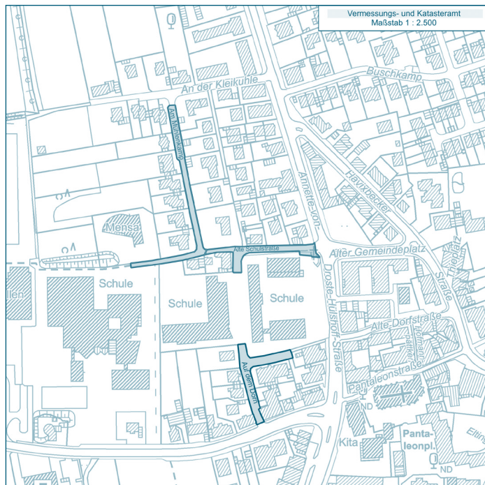
Übersichtsplan Nr. 1
